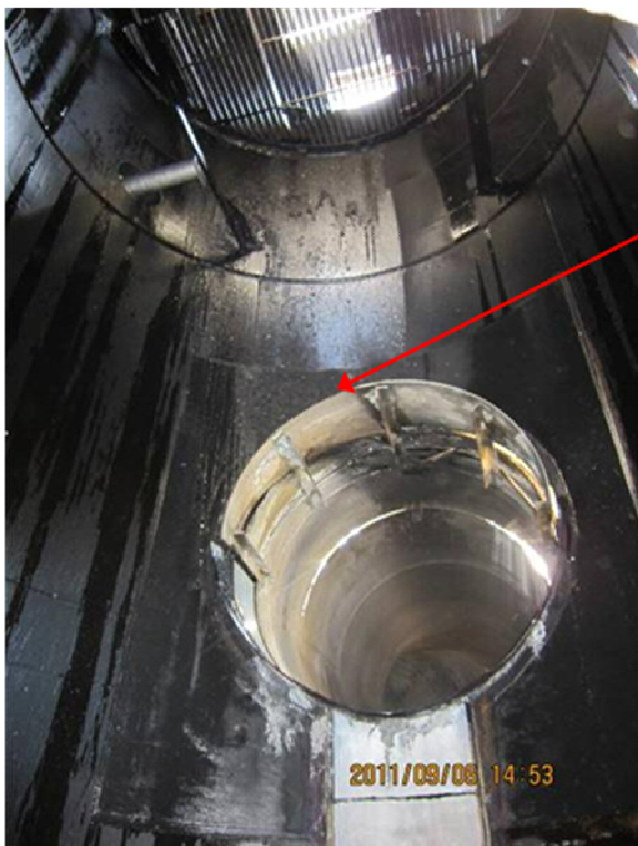
TCA内部 入口煙道 内壁 全面ゴムライニング4mm厚
