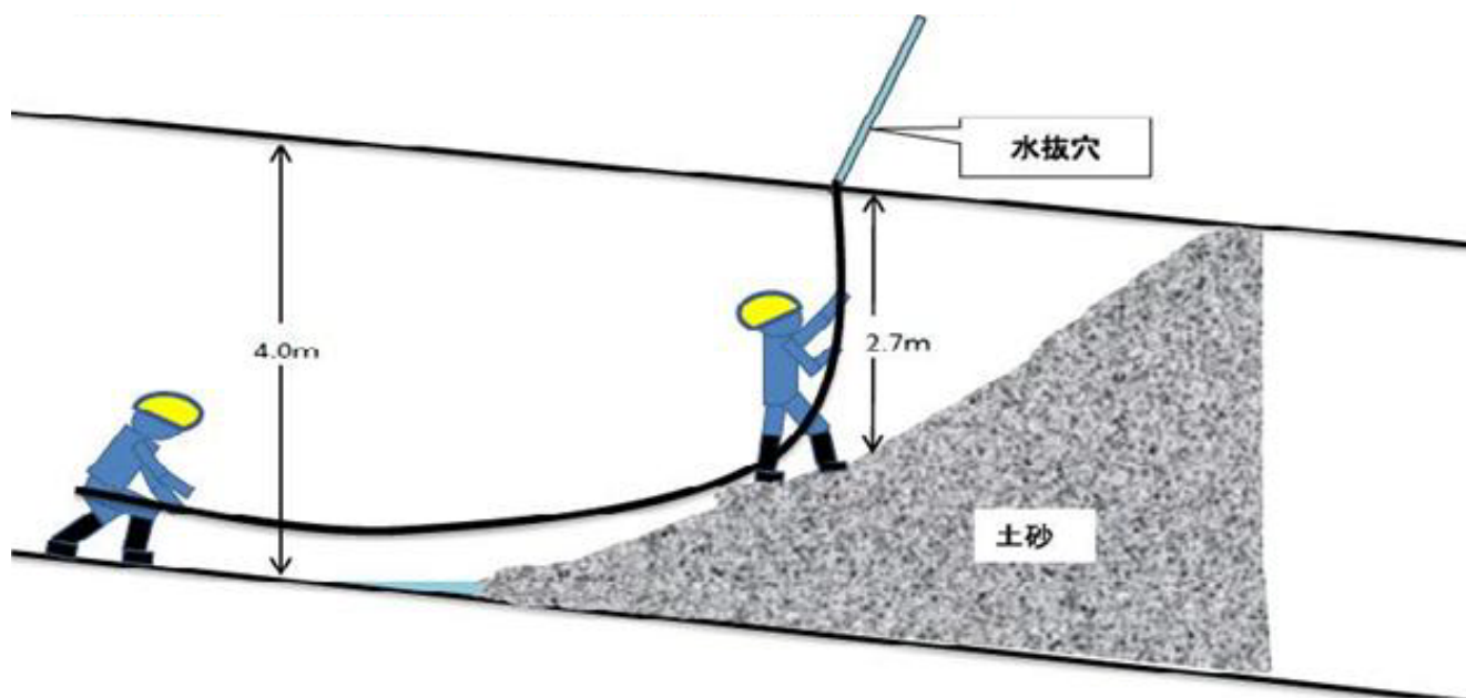
坑内 - 340m 平面図
