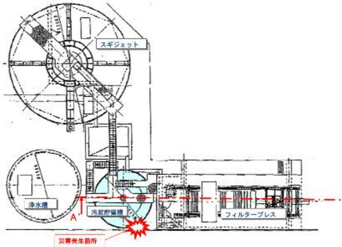
汚水処理施設平面図
