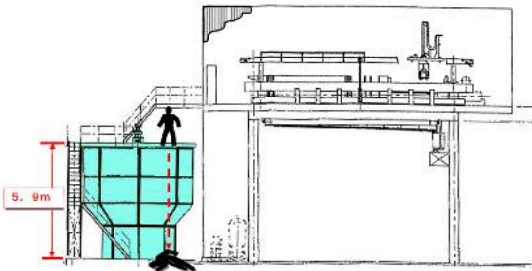
A-A' 汚水処理施設断面図
